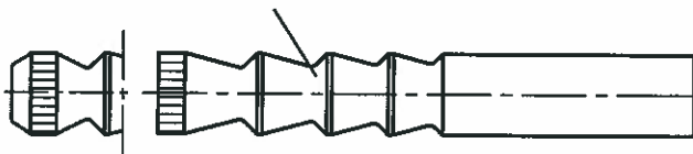
Anchor rod VMZ-IG 2)
